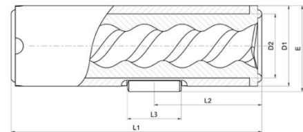
D1 = Ø 14,95 mm L1 = 46,50 mm L3 = 10,00 mm D2 = Ø 11,90 mm L2 = 19,20 mm E = 15,95 mm
